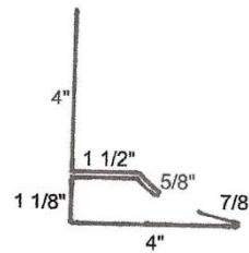
S. S. SW Flashing
