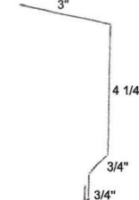
Mini Outside Corner*
