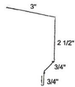
3X4 Eave
