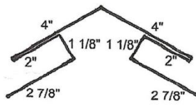
S. S. Hip Trim
