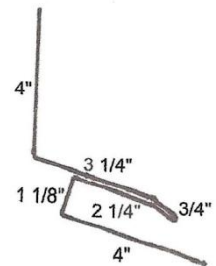
S. S. EW Flashing
