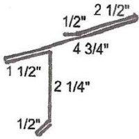
S. S. Drip Edge (Option 1)
