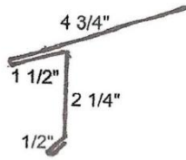
S. S. Drip Edge (Option 2)
