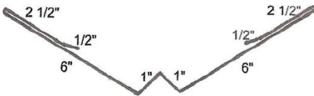
S. S. 20" Valley*
