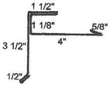
S. S. Rake*
