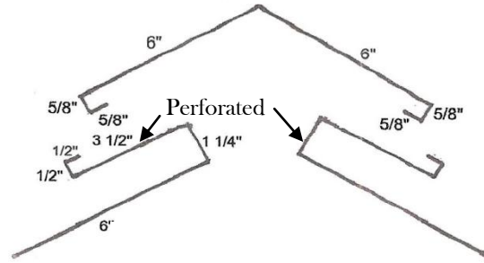
S. S. SW Flashing
