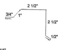
Mini Residential Rake*
