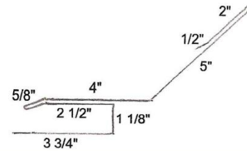
S. S. Lower Gambrel
