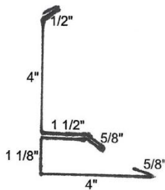
S. S. Chimney SW
