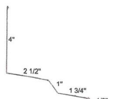
EW Flashing
