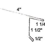
Drip Edge
