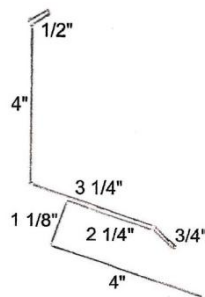
S. S. Chimney Lower
